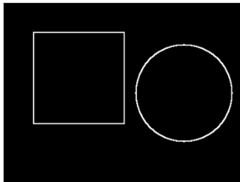
Sobel XY-axis
